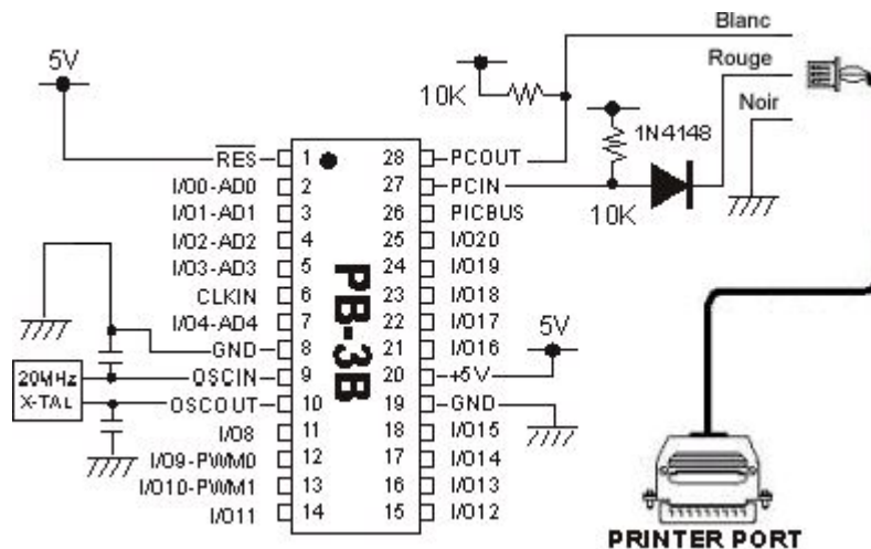
Schéma nécessaire à la mise en œuvre du "PICBASIC-3B"
